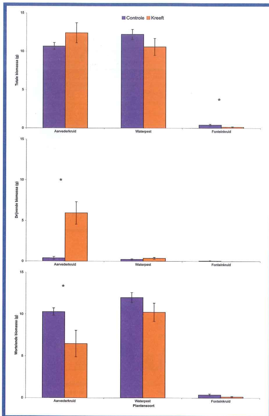
Afb. 1: Effecten van de Amerikaanse rode rivierkreeft op de waterplanten in de cilinders met en zonder kreeften. Significante effecten zijn aangegeven met een sterretje.
